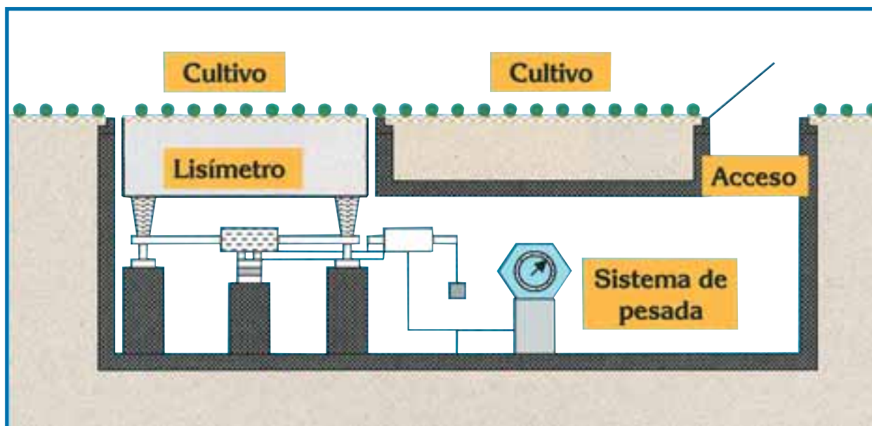
Figura n.º 1: Esquema de un lisímetro de pesada
